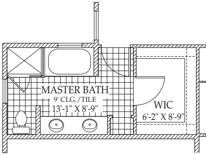
OPTIONAL MASTER BATH
